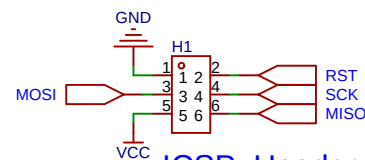
ICSP_Header
